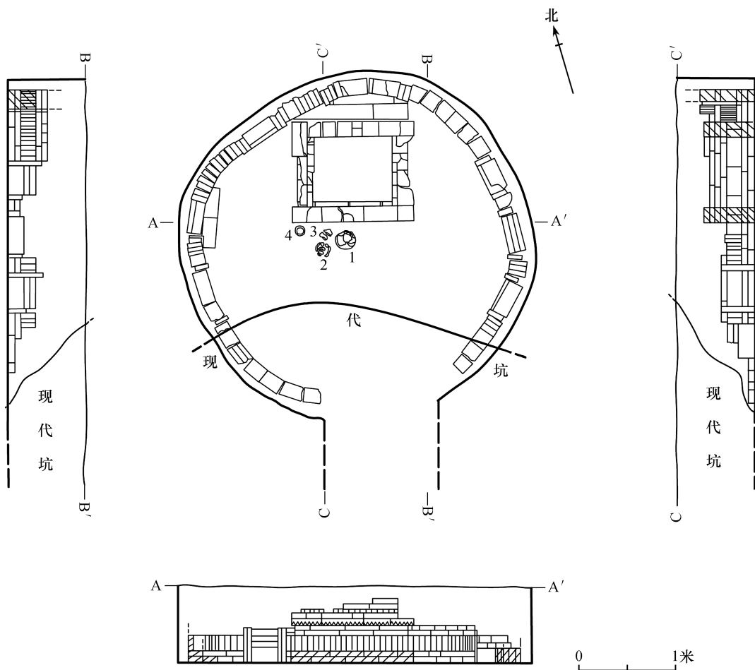
图七 M74平、剖面图
