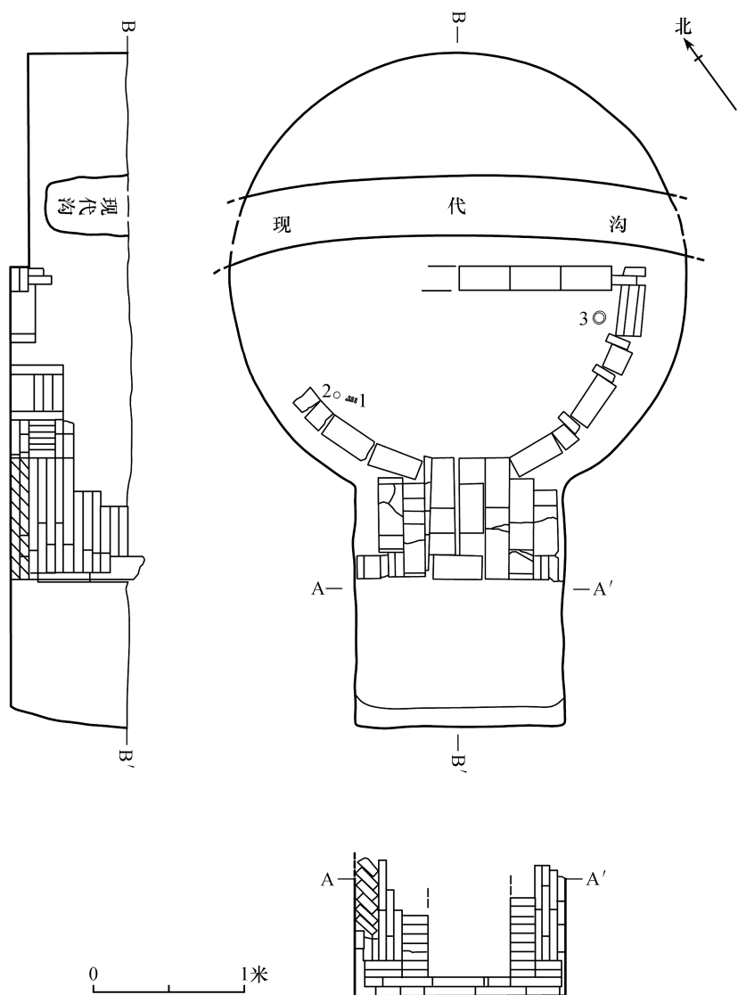
图五 M51平、剖面图
